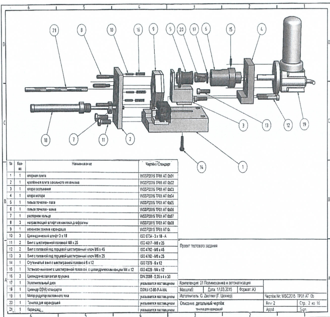
Рис 3. 3D модель сборки готового изделия «Точилка механизированная»
