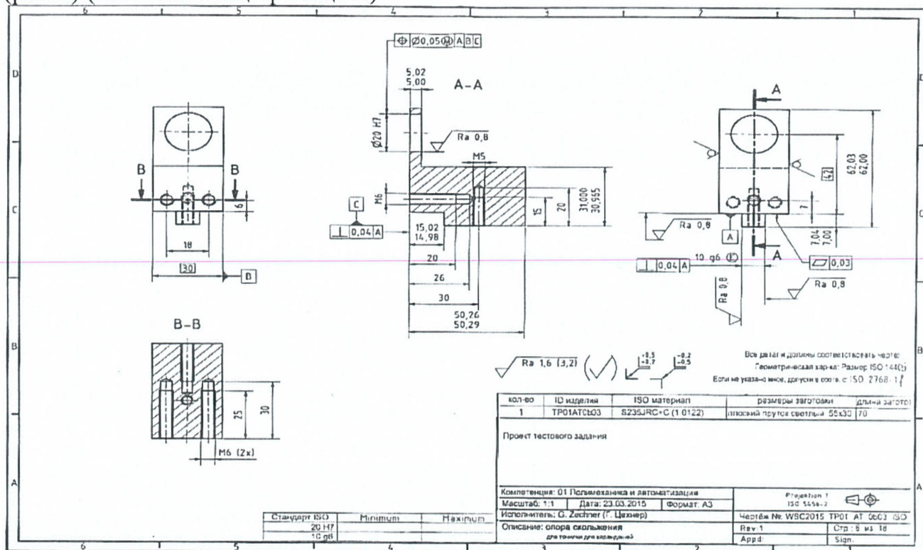
Рис 1. Чертеж детали поз. 3
